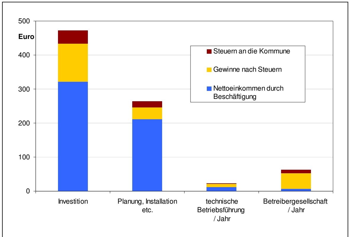
Abb. 3.7: Kommunale Wertschöpfung von PV-Großanlagen (Freiland), einmalige und jährliche Effekte, 2009
